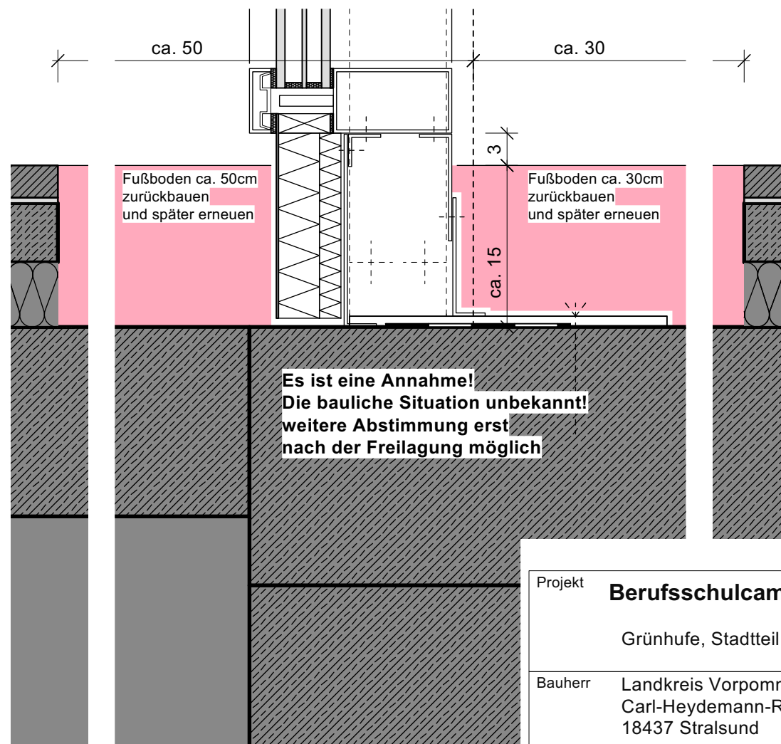
Detail 314-2 Vertikalschnitt PR 3-1 Erdgeschoss Eingang - Windfang (Ostfassade)
