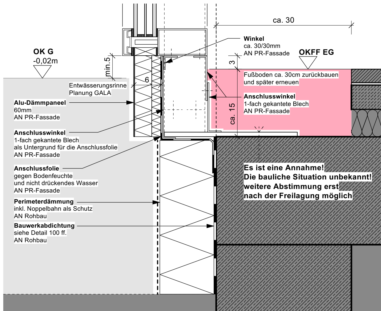
Detail 314-1 Vertikalschnitt PR 4-1 Erdgeschoss Eingang (Westfassade)
